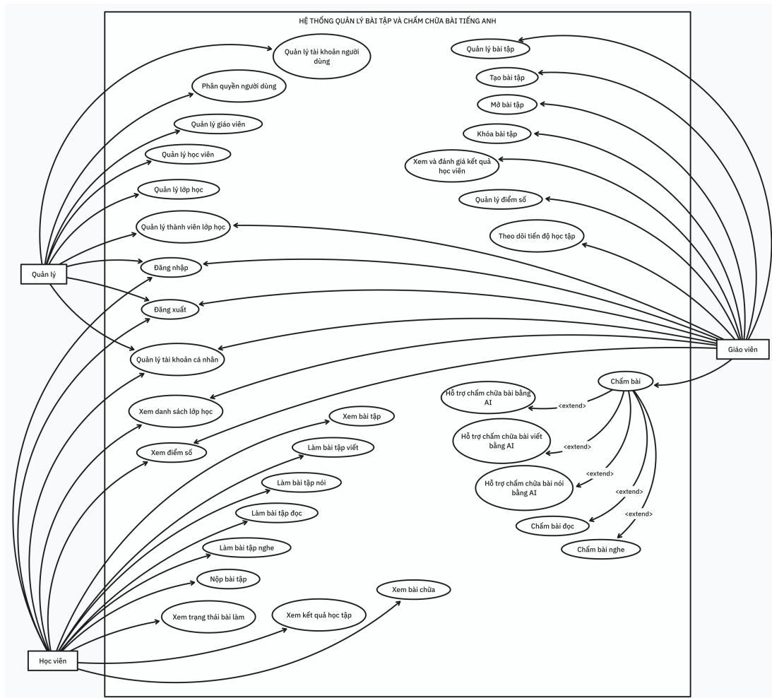
Hình 1: Sơ đồ ca sử dụng tổng quan
